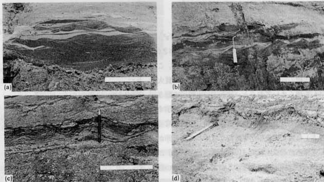
図1 新潟県小須戸町矢代田の兔谷層中のウェーブリップル。(a)ウェーブリップルの形成後、粘土層がこれを覆っている。形成時期が2~3回あることが分かる。(b)リップルの直上はシルト層である。(c)中粒~粗粒砂のウェーブリップル。(d)波長80cm~100cmのグラベルデューン。
