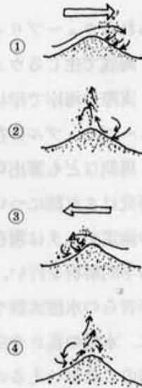
図11 ウェーブリップルの成長
