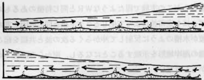
図10 底面の砂の移動
