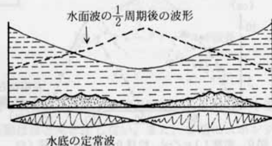
図6 水槽でできるウェーブリップルの全体像。水面の定常波の節の部分が波長、波高がともに最大で、砂も集積する。
