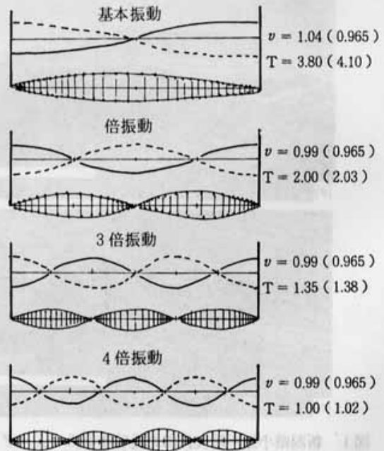
図4 基本振動～4倍振動の水面と水底の定常波の腹および節の位置。
