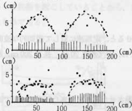
図7 水深12.5cm(上)と水深6.5cm(下)のときの倍振動での比較。黒丸はリップルの間隔(波長)棒線は底面からのリップルの高さ。
