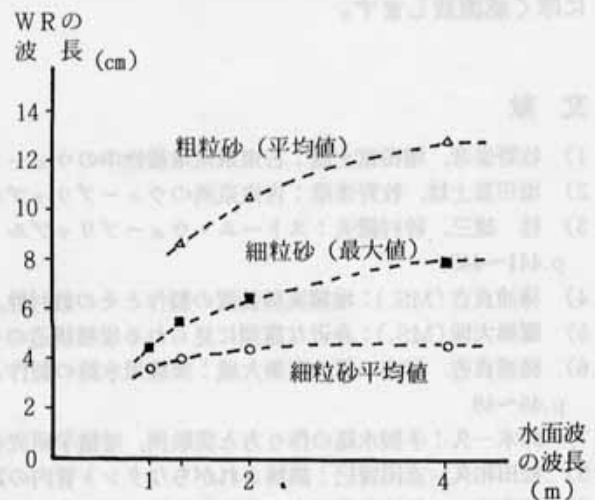
図13 水面波の波長とWRの波長の関係
