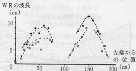
図9 密度1.1g/cm 3 , 粒径0.75mmの火山灰(白丸)と密度2.5g/cm 3 , 粒径0.75mmの粗粒砂(黒丸)の場合
